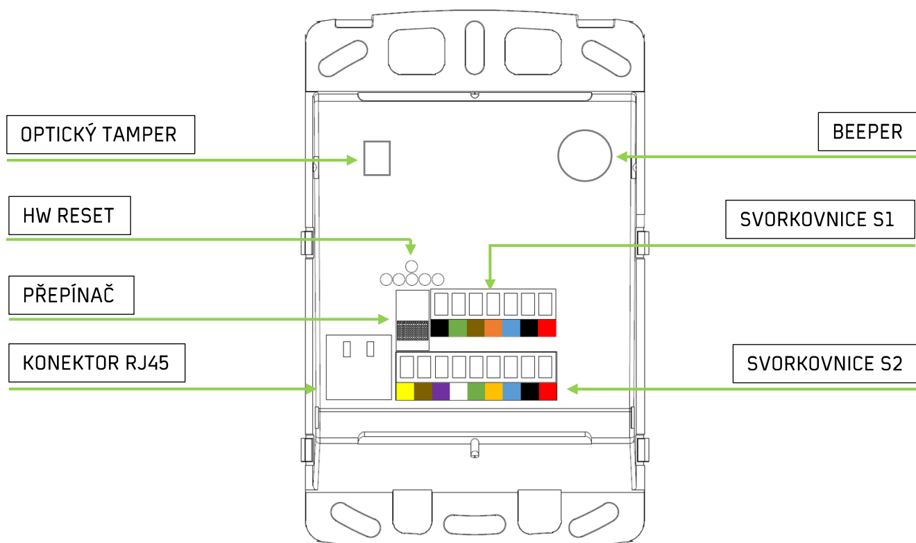
Obr. 9: Funkční prvky
