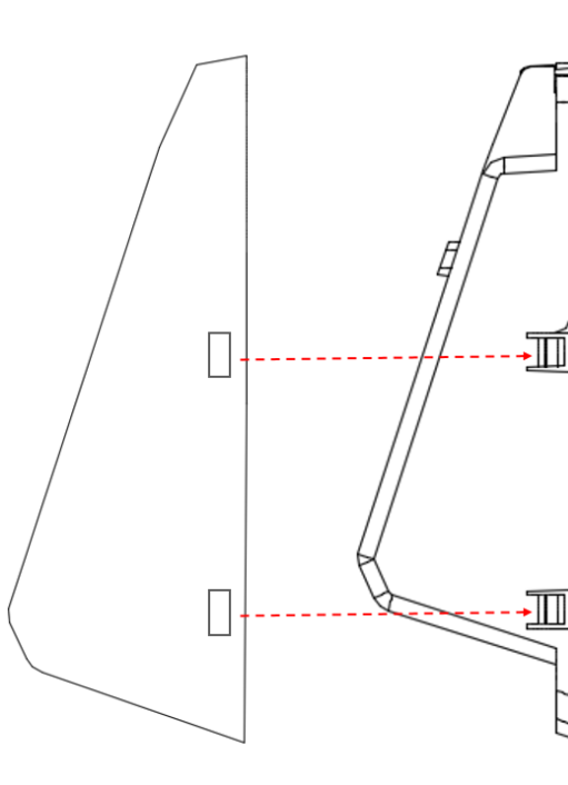
Obr. 2: Nasazení krytu
