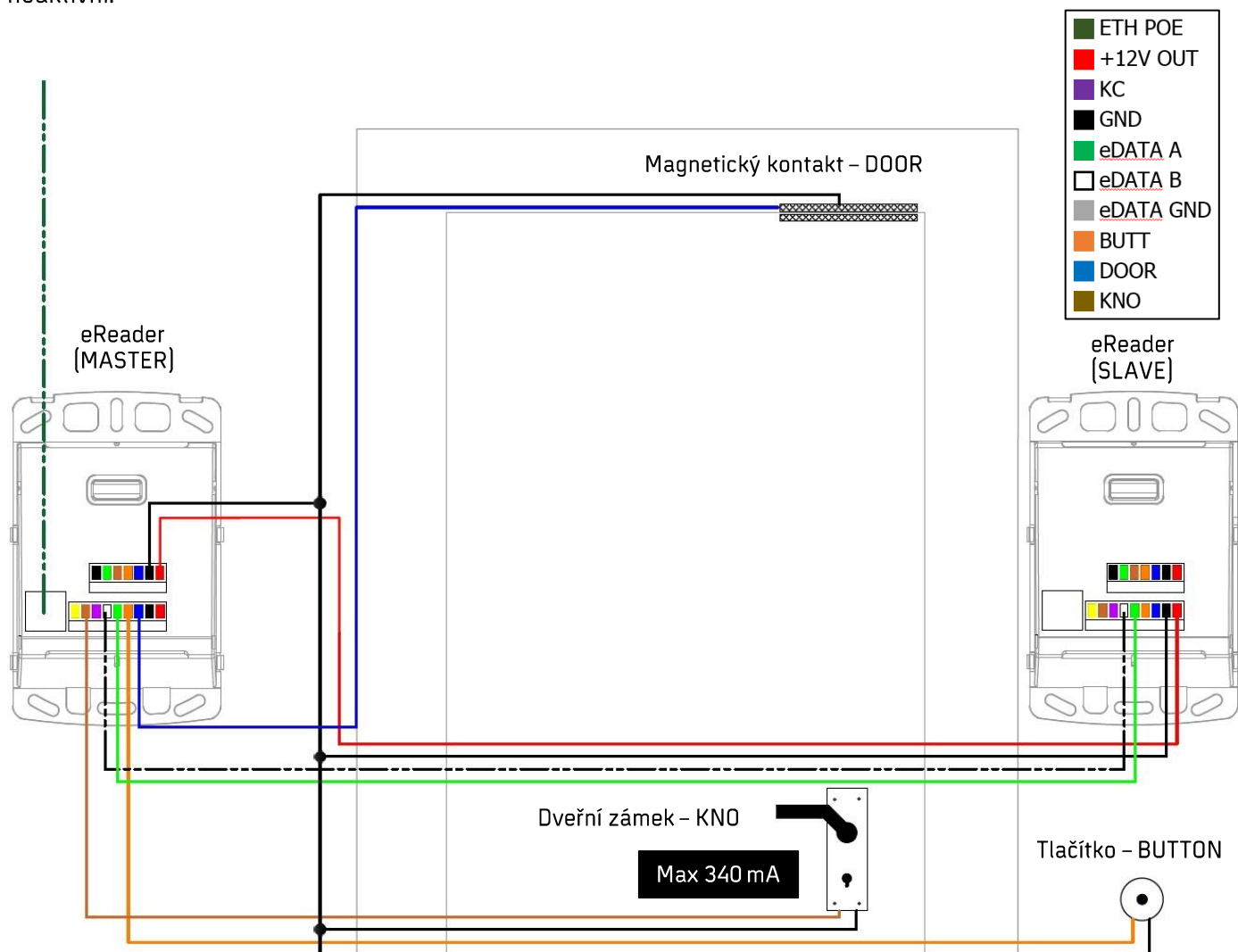
Obr. 384: Zapojení systému – varianta 3
