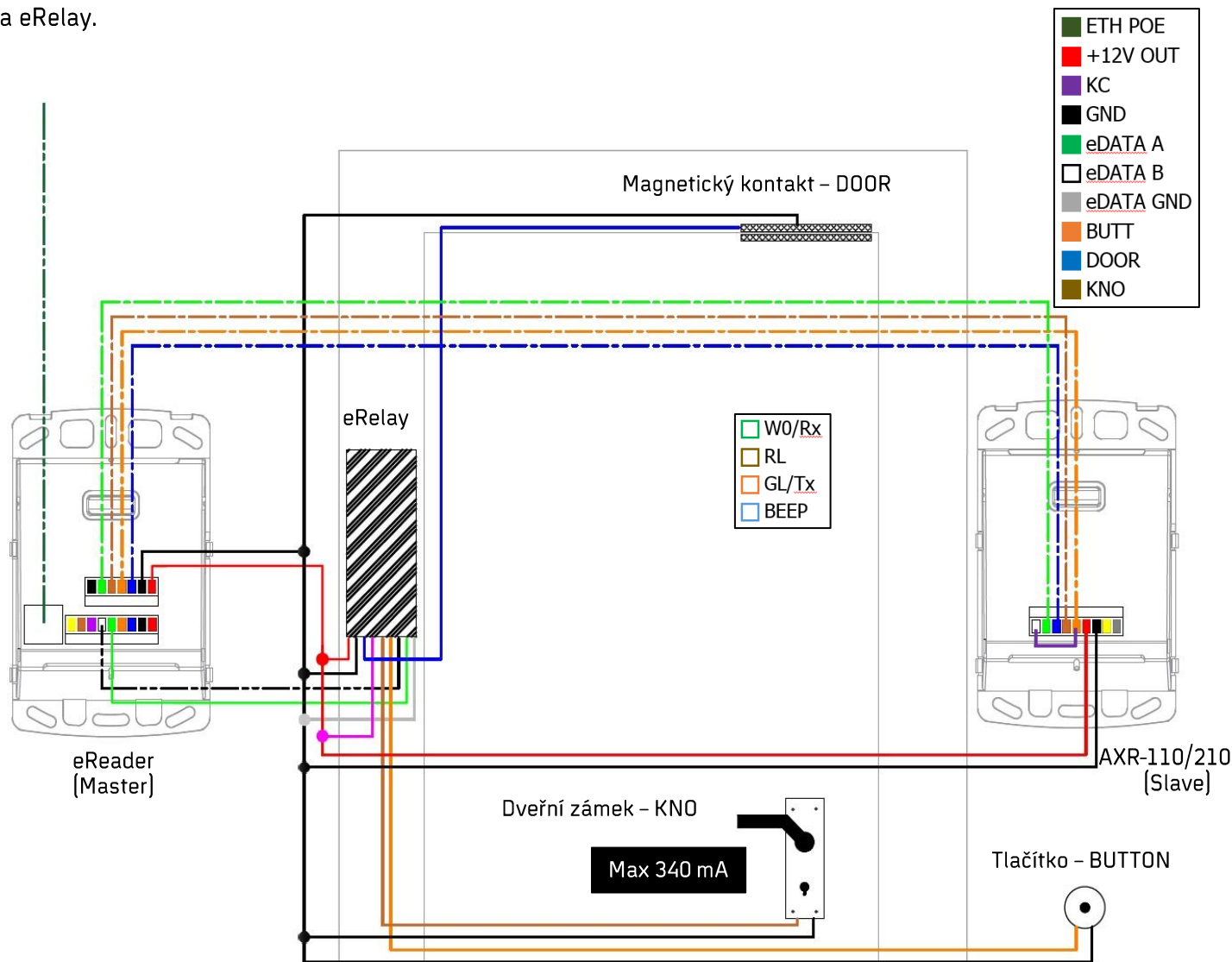
Obr. 373: Zapojení systému – varianta 2
